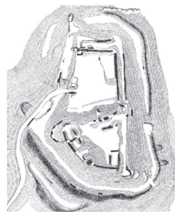
Plan założenia zamkowego twierdzy Edelštejn, P. Kouřil, D. Prix, M. Wihoda: Hrady českého Slezska , AÚ AV ČR Brno, 2000
