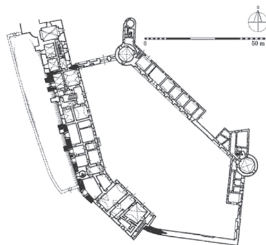
Plan założenia zamkowego P. Kouřil, D. Prix, M. Wihoda: Hrady českého Slezska , AÚ AV ČR Brno, 2000
